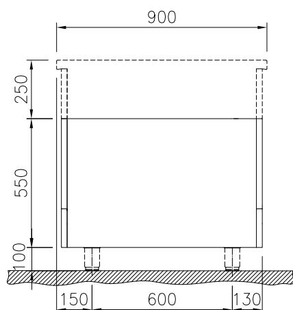
Zij aanzicht
